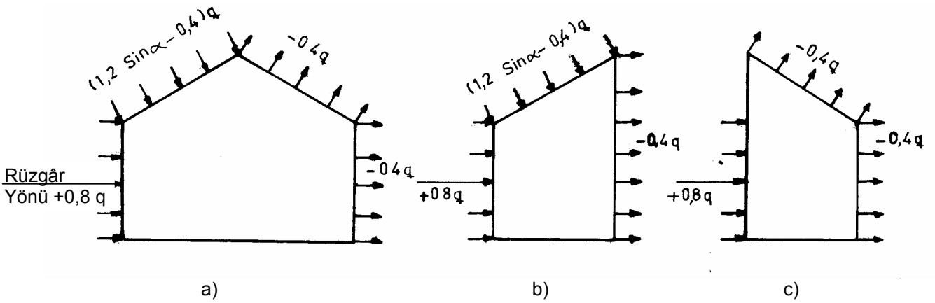
ŞEKİL 1 - Planda Kare Kesitli ve Eğik Çatılı Kapalı Yapılarda Rüzgar
